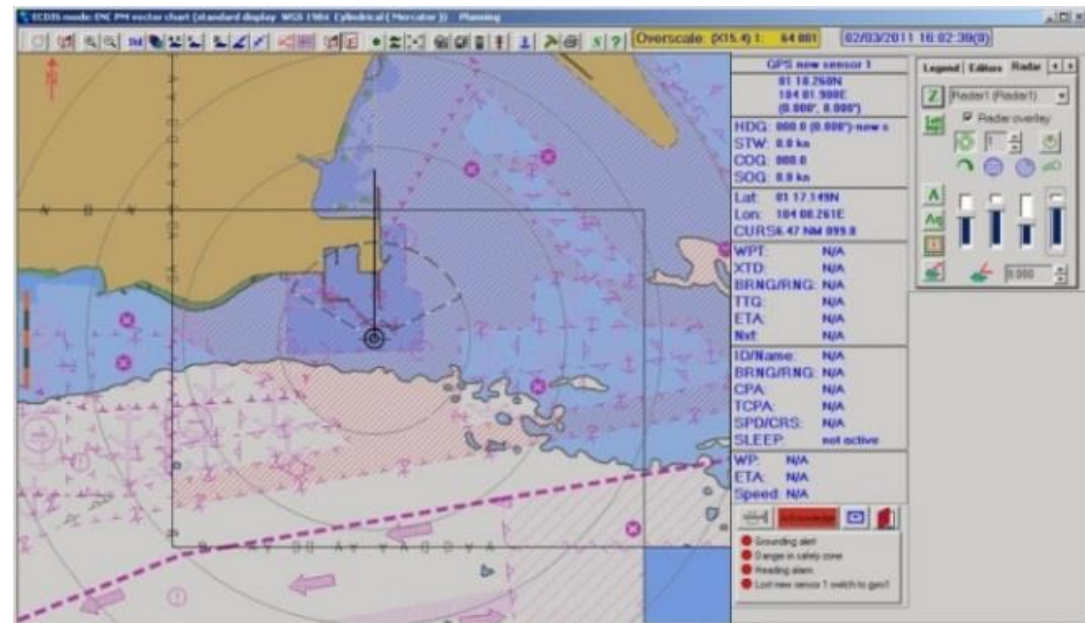
ECDIS Display
